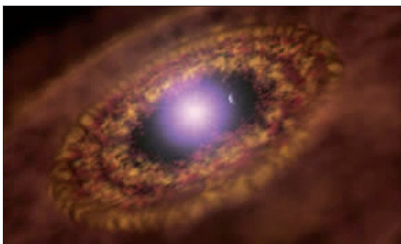
最“年幼”的行星和它周围的原行星盘
