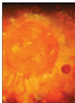
最年幼行星年仅1000万年
