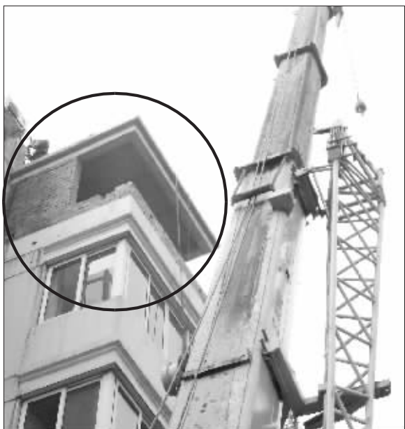
机械化拆除钢混违建
