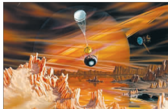
艺术家绘制的土卫六提坦上连绵的沙丘和山脉
