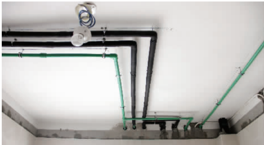
水管顶部排布要横平竖直，用吊筋固定，热水管及循环水管进行保温处理
