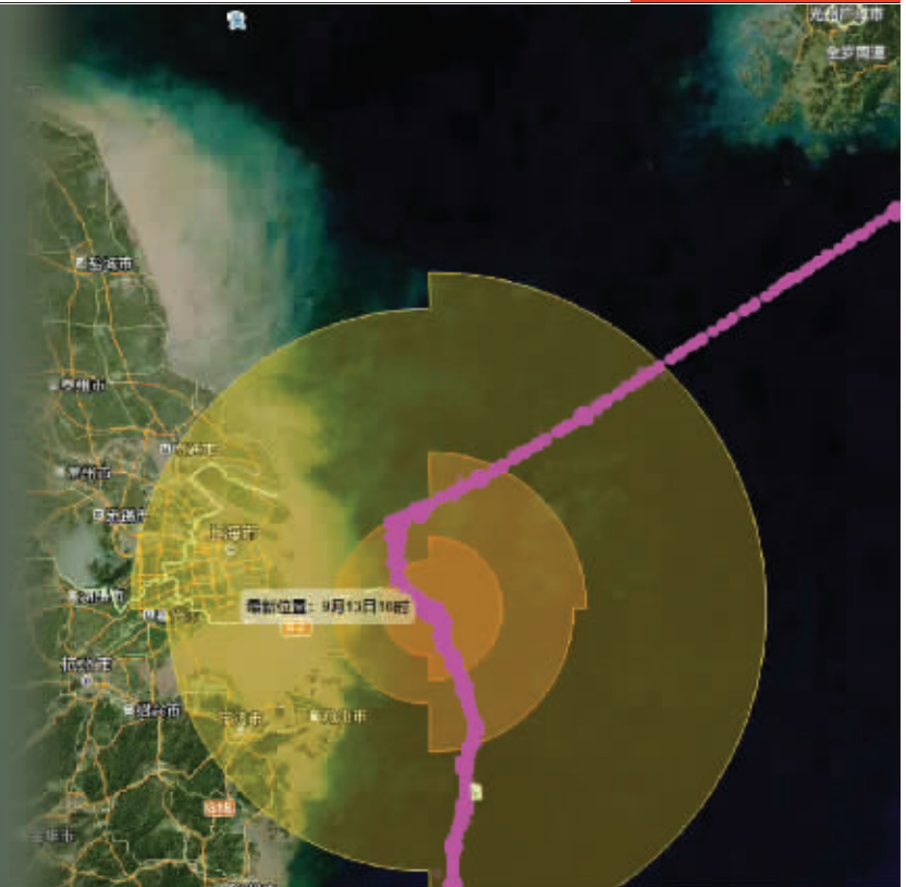
“灿都”未来路径概率预报图(中央气象台)
